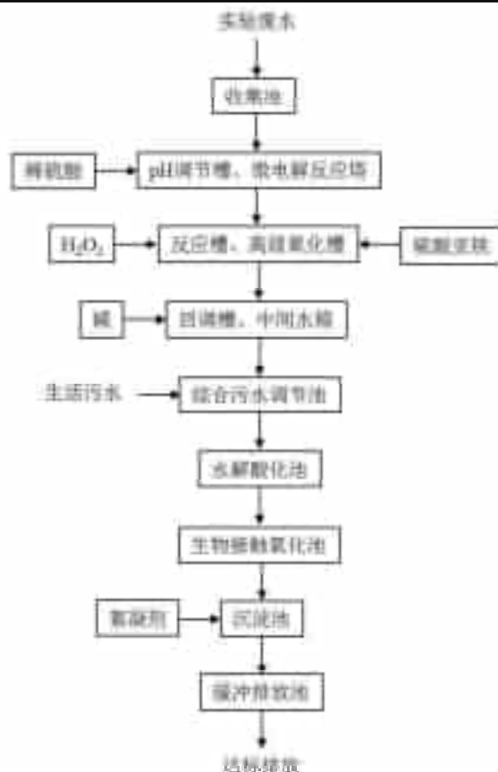
图 4-2 园区一、二期污水处理站工艺流程图
