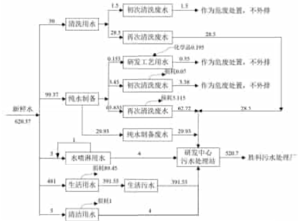
图 2-8 现有项目水平衡图 (单位: m³/a)
