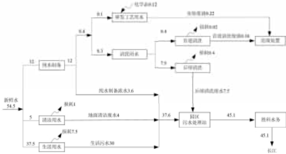
图 2-1 本项目水平衡图 (单位: \text{m}^3/\text{a} )
