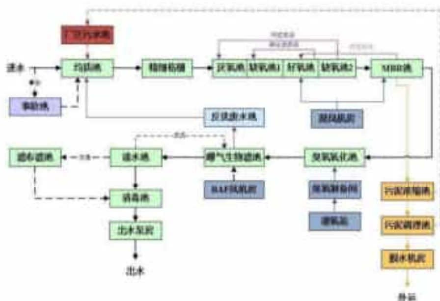
图 4-3 南京胜科水务有限公司一期工程流程图
