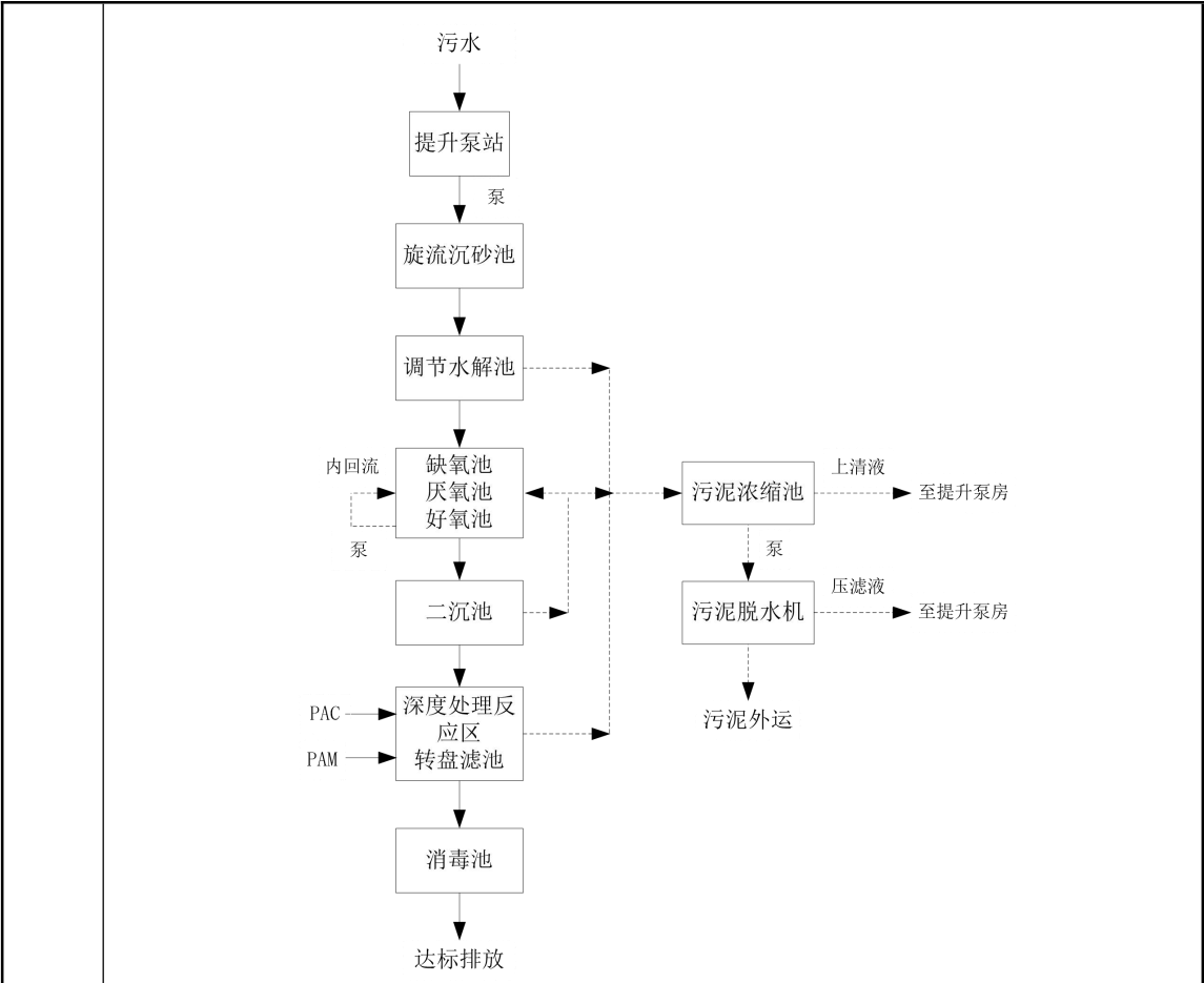
图 4-2 盘城污水处理厂工艺流程图
